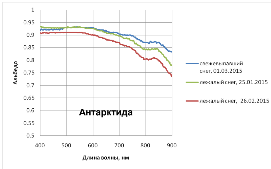
Спектры альbedo снежного покрова в Антарктиде
