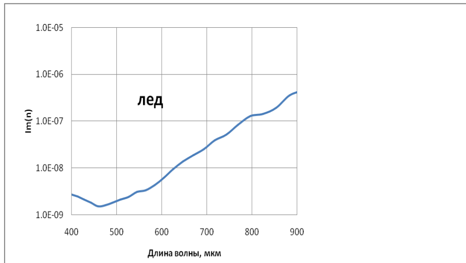
Спектры мнимой части показателя преломления Im(n) льда
