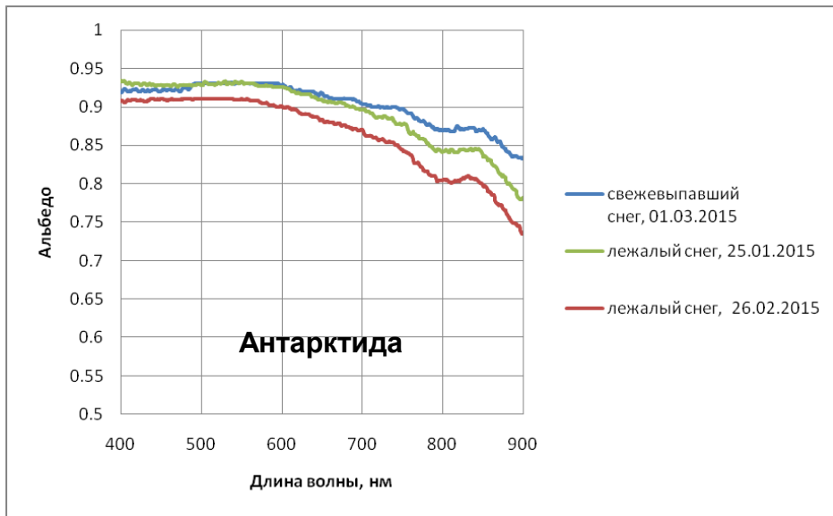
Спектры альbedo снежного покрова в Антарктиде и Беларуси
