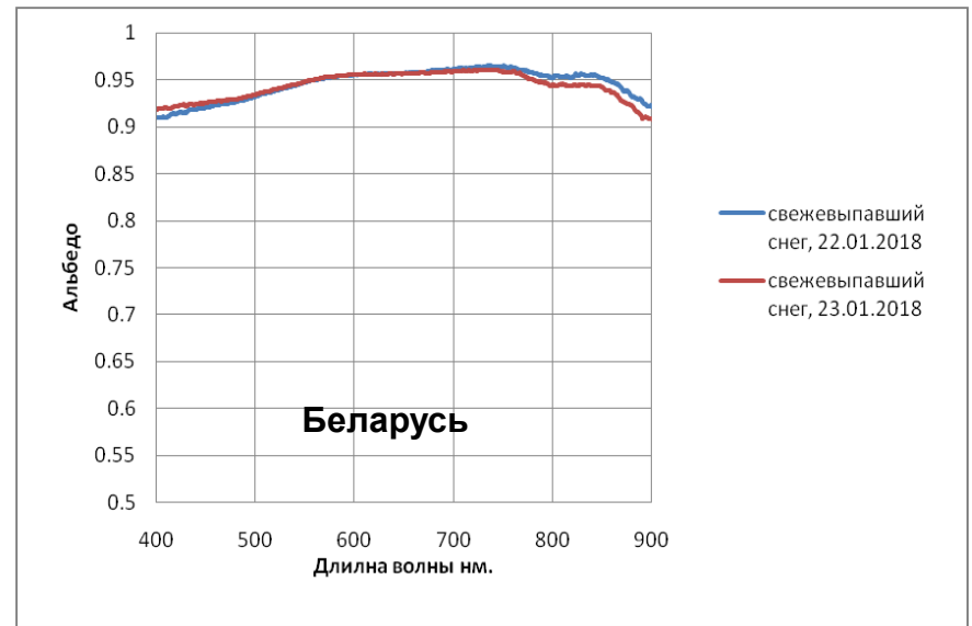
Спектры альbedo снежного покрова в Антарктиде и Беларуси
