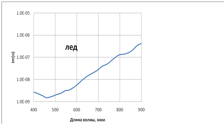
Спектры мнимой части показателя преломления Im(n) сажи и льда
